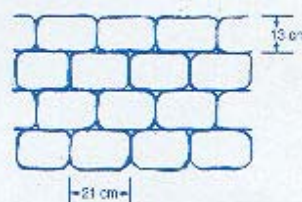
ADOQUIN ALHOHADILLADO
